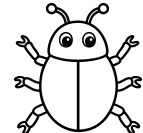
bug
