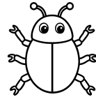
bug
